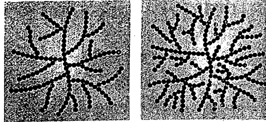
Glycogen
